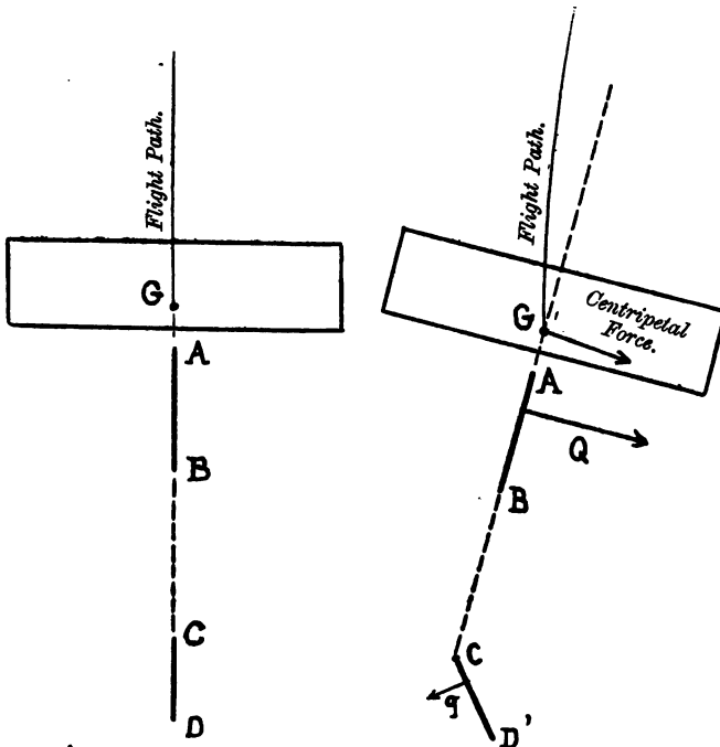
FIG. 77.—Plan.
